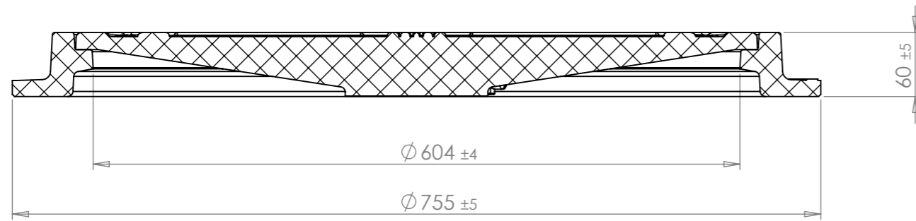
ŘEZ A-A MĚRITKO 1 : 5
