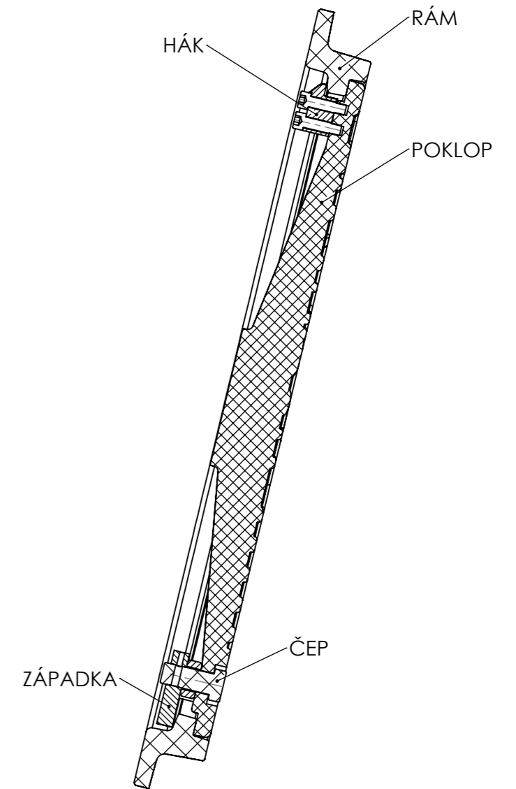
ŘEZ B-B MĚRITKO 1 : 5
