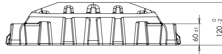
PRŮTOČNÝ PRŮŘEZ 80 203 mm 2
